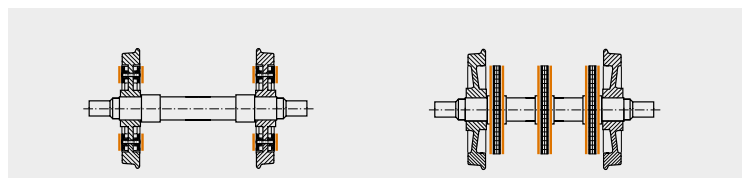
Brake discs
